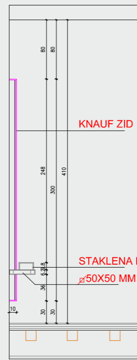
PRESJEK B-B M 1:50
