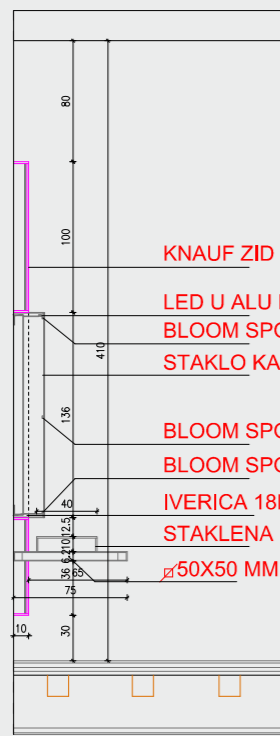
PRESJEK A-A M 1:50
